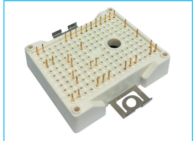
Rectifier+Brake+Inverter
